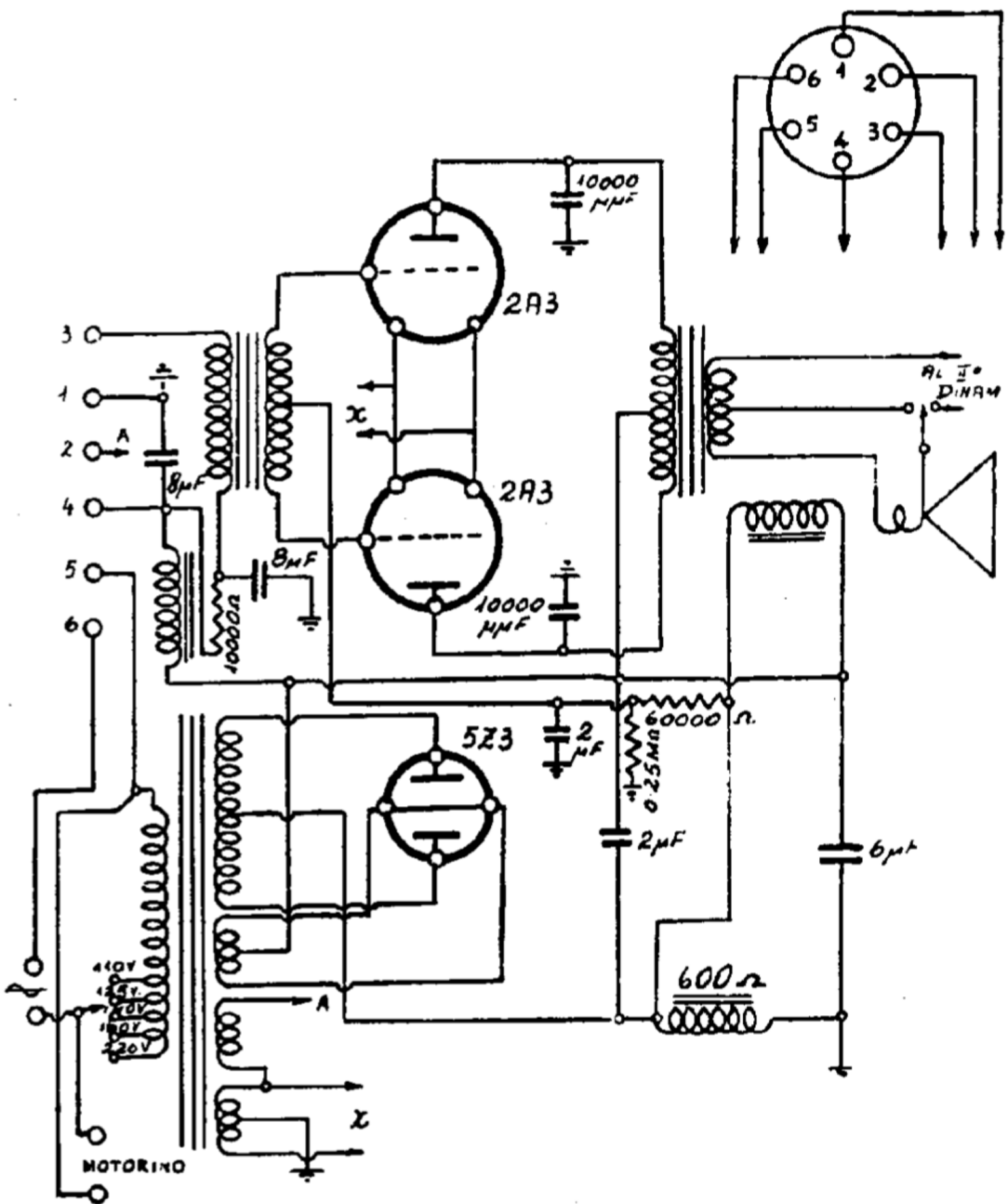
RADIO SAFAR. — Parte amplificatrice b. f. e alimentatrice dei modelli « 53 e 73 ».
